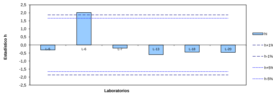
Estadístico de consistencia inter-laboratorio de Mandel Frecuencia 5000 Hz
