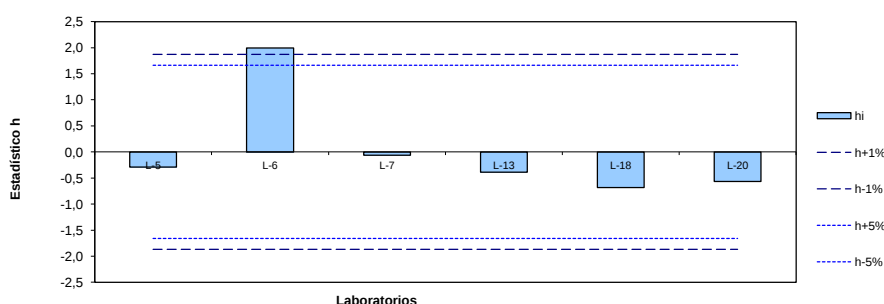
Estadístico de consistencia inter-laboratorio de Mandel Frecuencia 4000 Hz
