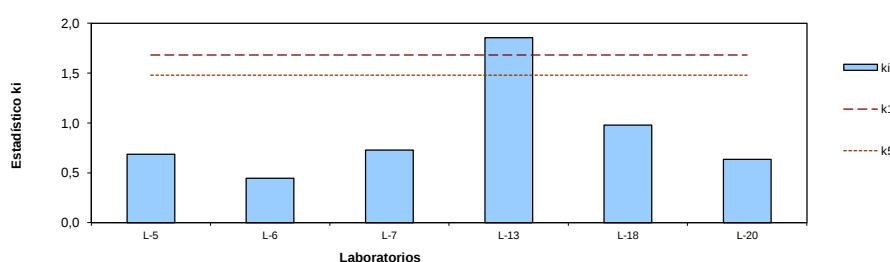
Estadístico de consistencia intra-laboratorio de Mandel Frecuencia 4000 Hz
