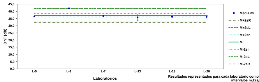
Representación de los valores de cada laboratorio con los límites de dos desviaciones Frecuencia 5000 Hz
