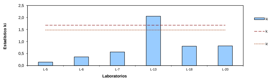
Estadístico de consistencia intra-laboratorio de Mandel Frecuencia 5000 Hz
