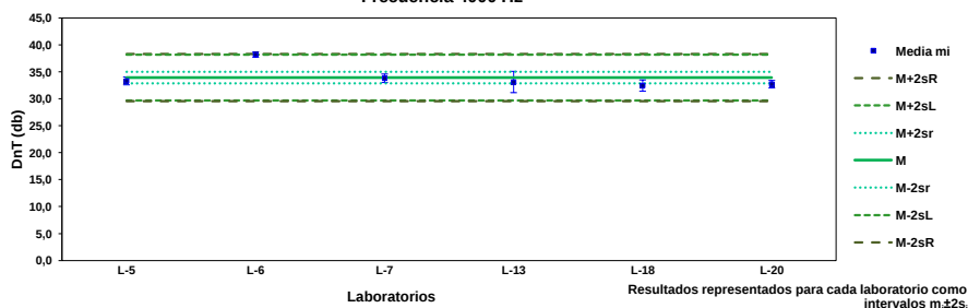
Representación de los valores de cada laboratorio con los límites de dos desviaciones Frecuencia 4000 Hz
